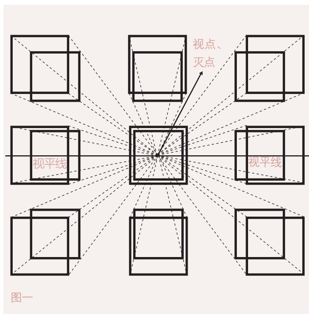
▲ 一点透视
