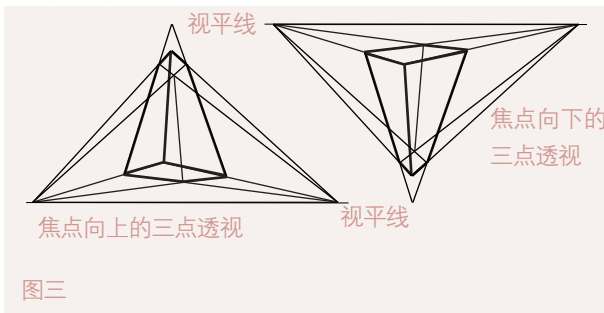
▲ 三点透视
