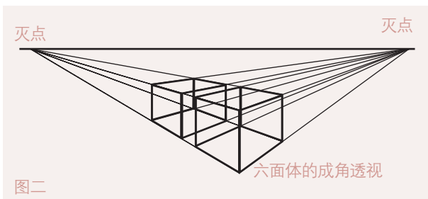
▲ 两点透视
