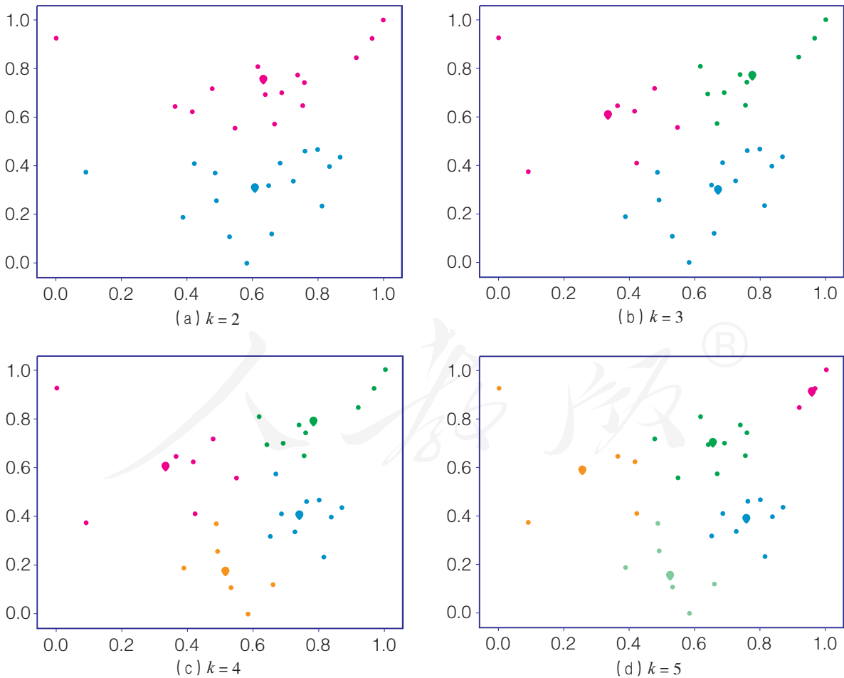
图2.4.5 k 的取值依次为2、3、4、5时得到的聚类图
