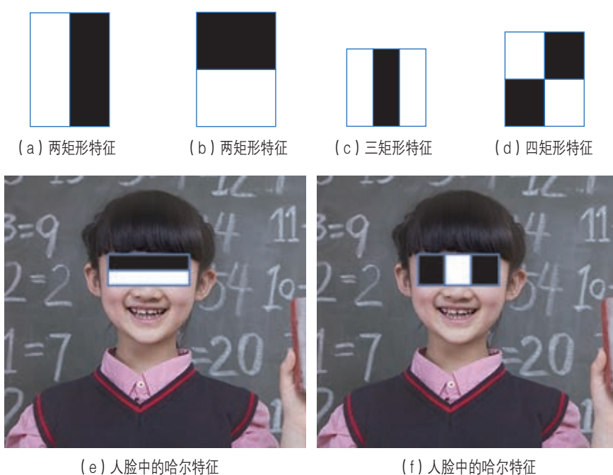
图3.1.7 哈尔特征
