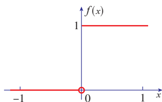
图2.5.4 函数 f(x) 的图像
