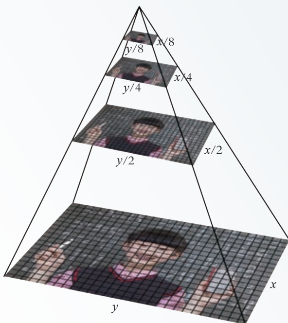
图 3.1.10 图像金字塔
