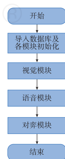
图 3.5.12 智能陪伴机器人的主程序流程图
