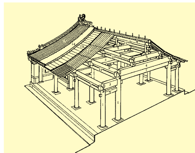
中国古代建筑主要屋顶样式示意图
